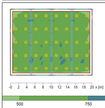
Anordnung der Leuchten im Saal und Lichtberechnung
